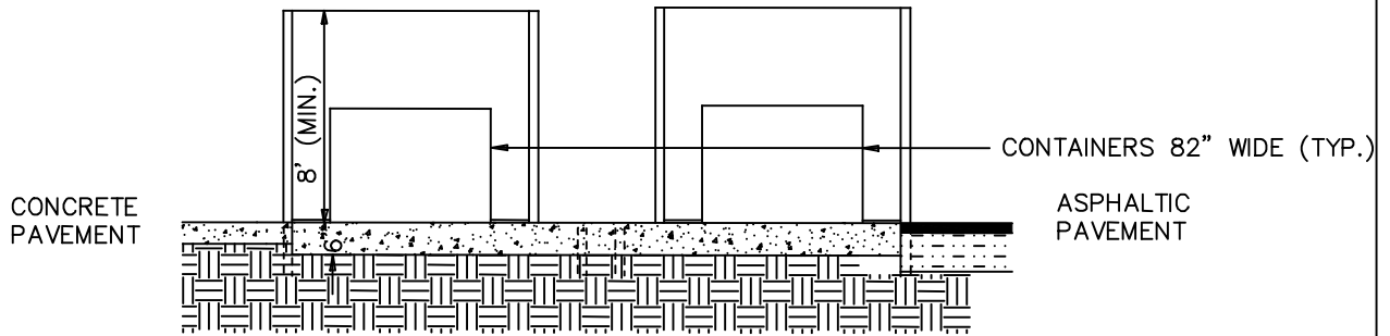
ELEVATION
